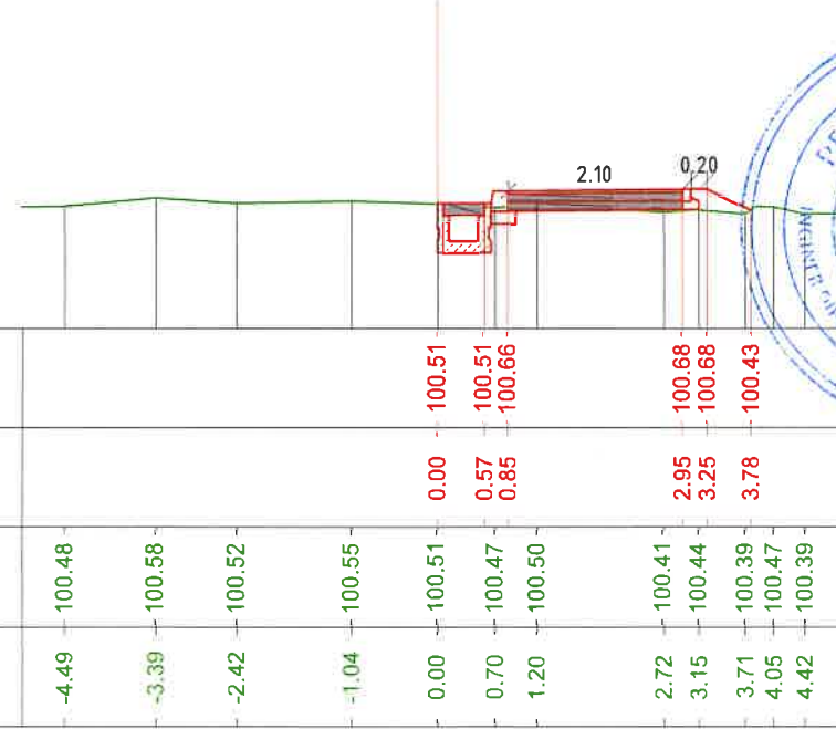
Piste biciclete Roata de Jos - km 1+680.000
