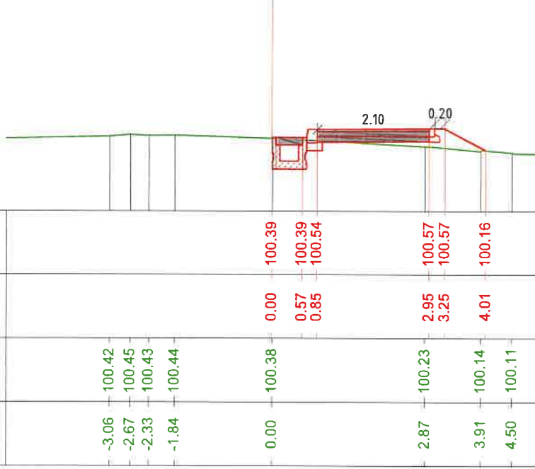
Piste biciclete Roata de Jos - km 1+660.000
