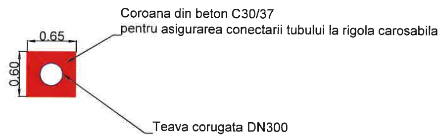
SECTIUNE TRANSVERSALA B-B
