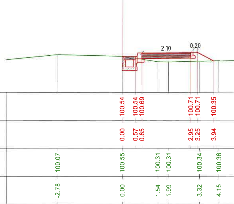
Piste biciclete Roata de Jos - km 1+460.000
