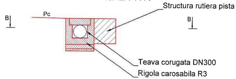
SECTIUNE TRANSVERSALA A-A
