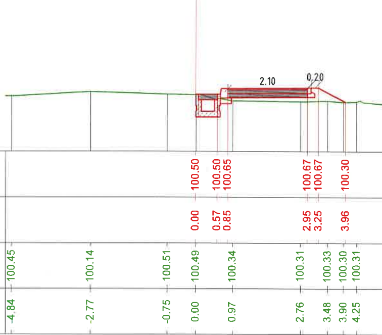
Piste biciclete Roata de Jos - km 1+440.000
