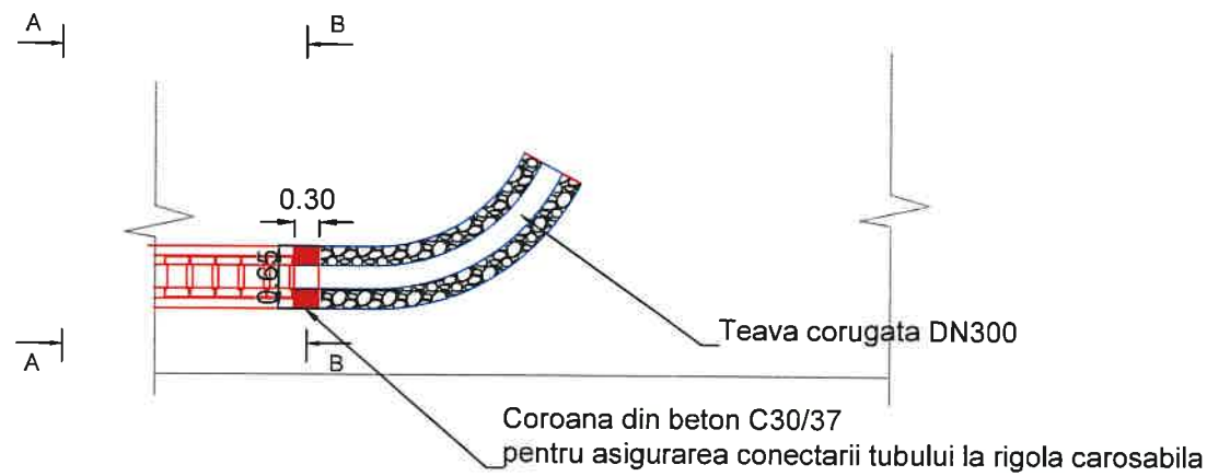
VEDERE IN PLAN B-B
