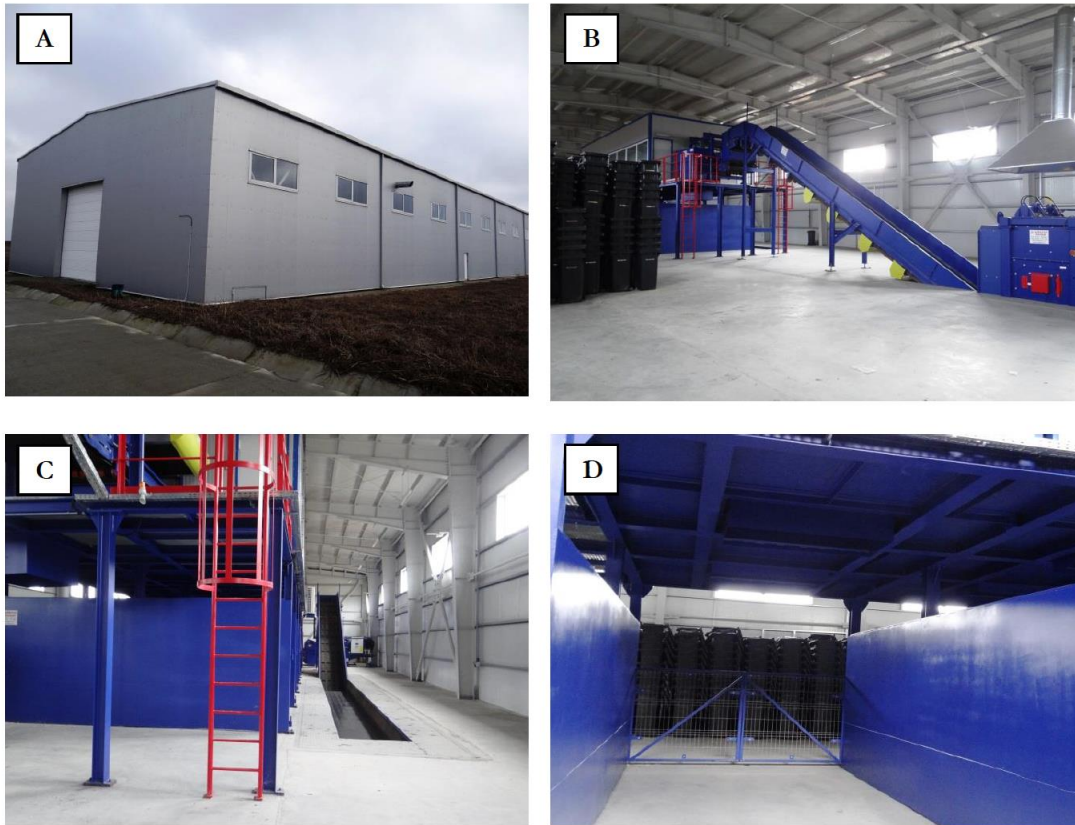
Figura 2 Stația de sortare – (A) Hala de sortare; (B) Stația de sortare; (C) Banda transportoare; (D) Buncăr material sortat
